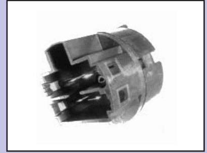
JK491 INTERRUPTOR DE CONTACTO ALFA - FIAT - LANCIA PUNTO II - BRAVO - MAREA - PALIO - Y
