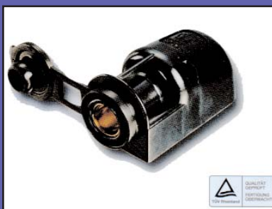
028003 BASE TOMA CORRIENTE UNIVERSAL DIAMETRO 18,5 TIPO DIN/ISO 4165 CON TAPA - 16 A. A 12-24V-SUPERFICIE
