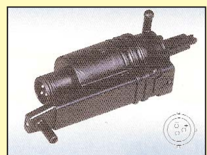
HS-277B AUDI - 12 V BOMBA LAVAPARABRISAS 2400 ml/min NUEVA
