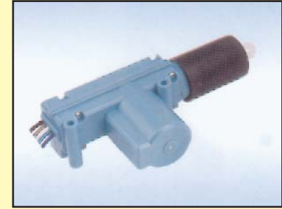
HS-714 B MOTOR BLOCAPUERTAS 5 CABLES 12V
