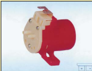
HS-212A UNIVERSAL - PEUGEOT - LADA 12 v 1320 ml/min
