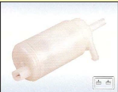
HS-316A SCANIA - 24 V BOMBA LAVAPARABRISAS 1200 ml/min NUEVA
