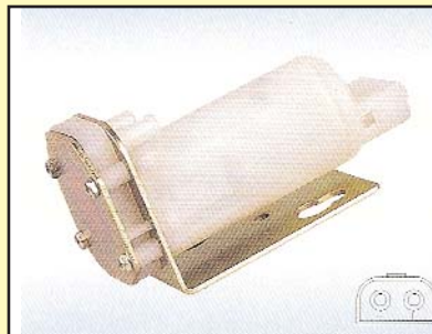
HS-316C VOLVO - 24 V BOMBA LAVAPARABRISAS 1200 ml/min NUEVA
