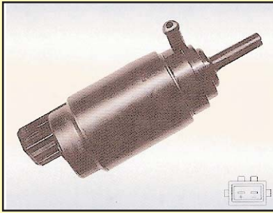
HS-232 SEAT - AUDI - VOLSWAGEN - 12 V LAVAPARABRISAS CONECTOR 2200 ml/min NUEVA
