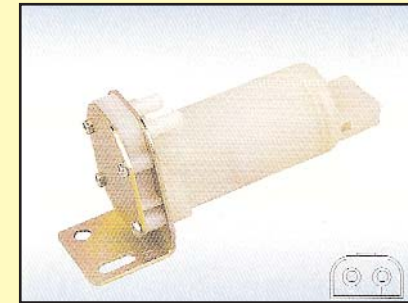
HS-316D VOLVO - 24 V BOMBA LAVAPARABRISAS 1200 ml/min NUEVA
