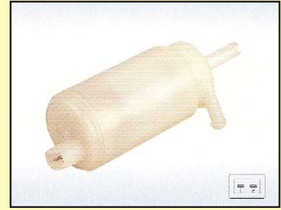
HS-288C MERCEDES - SCANIA - 24 V BOMBA LAVAPARABRISAS 2600 ml/min NUEVA
