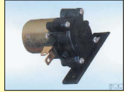
HS-211B24 UNIVERSAL - 24 V 1200 ml/min
