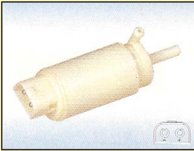
HS-288A SCANIA 24 V BOMBA LAVAPARABRISAS CON CONECTOR 1400 ml/m NUEVA
